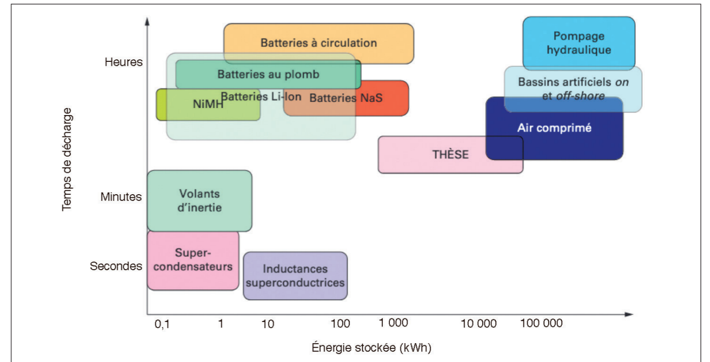
▲ Figure 15. Comparatif des performances de différentes technologies de stockage d'énergie. Source : Techniques de l'Ingénieur.
