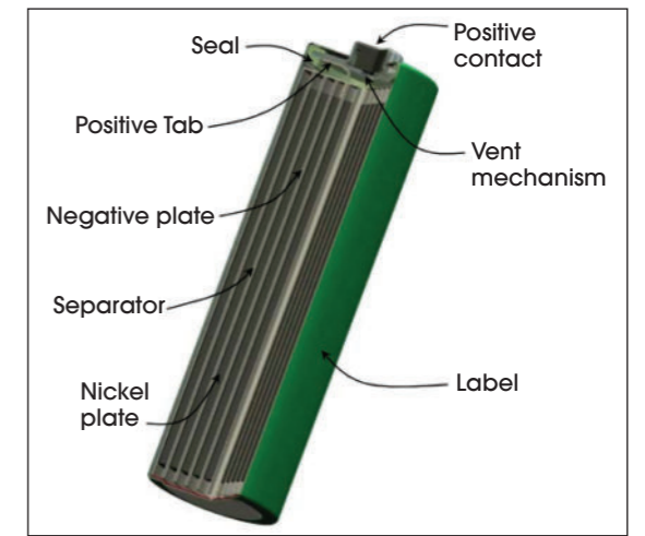
▲ Figure 4. Schéma d'une pile type nickel. Source : perma-batteries.com
