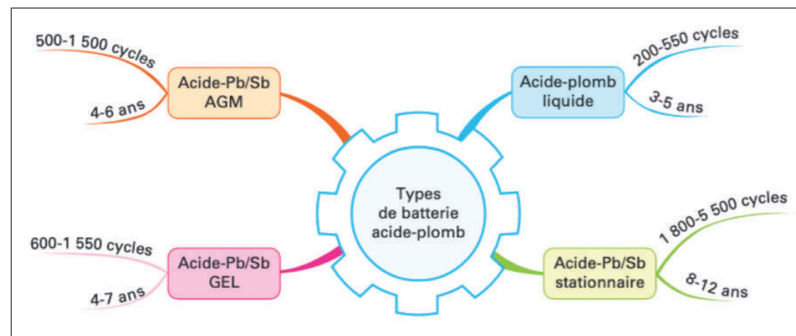
▲ Figure 3. Performances des batteries acide-plomb. Source : Techniques de l'Ingénieur.
