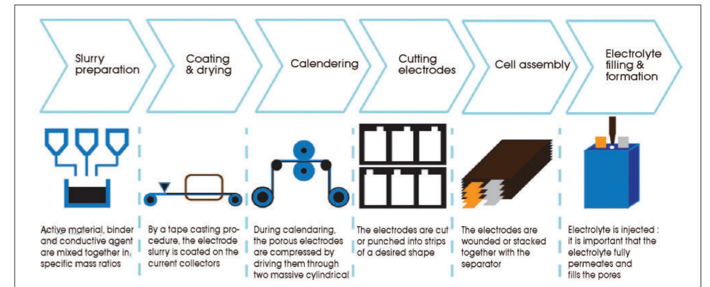
▲ Figure 10. Étapes de fabrication d'une batterie. Source : researchgate.net.
