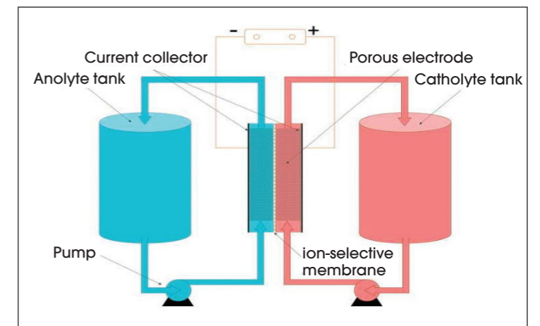
▲ Figure 16. Schéma d'une pile à écoulement.
