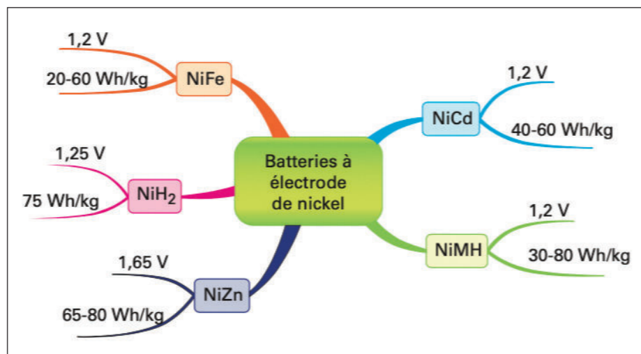
▲ Figure 5. Performances des batteries au nickel. Source : Techniques de l'Ingénieur.
