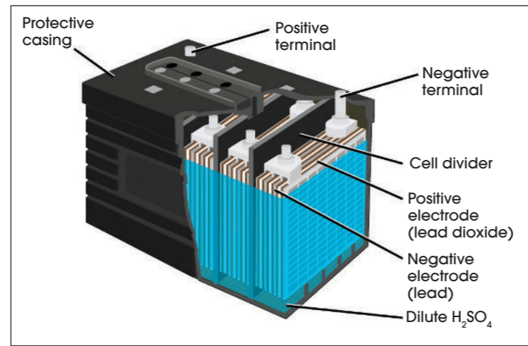
▲ Figure 2. Schéma d'une batterie acide-plomb. Source : Wikipédia.
