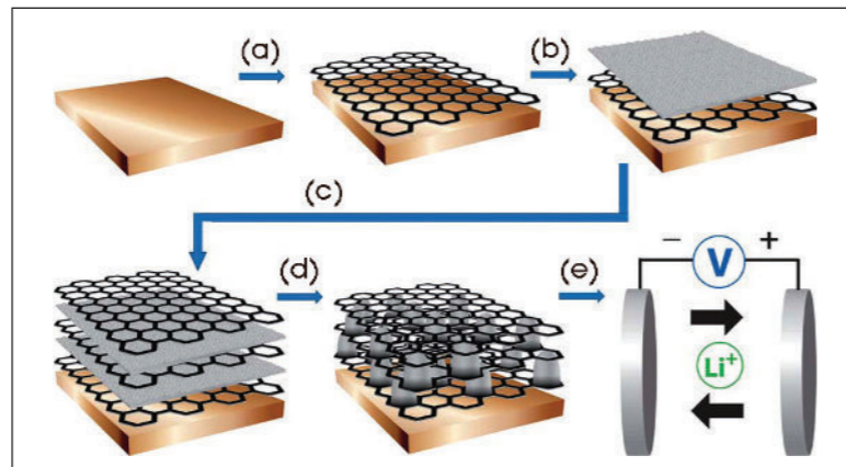
▲ Figure 12. Schéma d'assemblage d'une batterie au graphène. Source : Techniques de l'Ingénieur.
