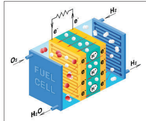
▲ Figure 17. Schéma d'une pile à combustible. Source : airbus.com.
